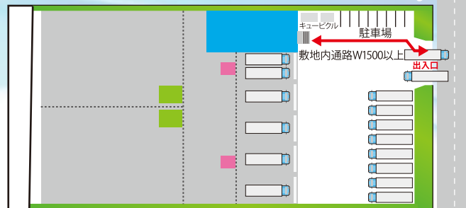
敷地図
